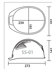
SS-01型寸法図
