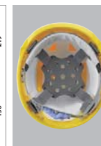
SS-19VRA内装 ●ラチェット式調整 ●タオルバンド ●スチロール
